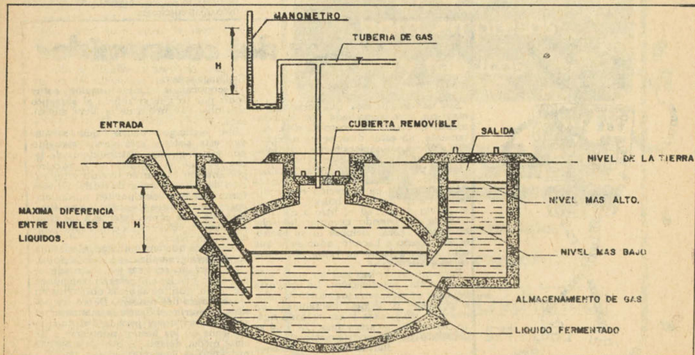
Planta de Bio Gas.
