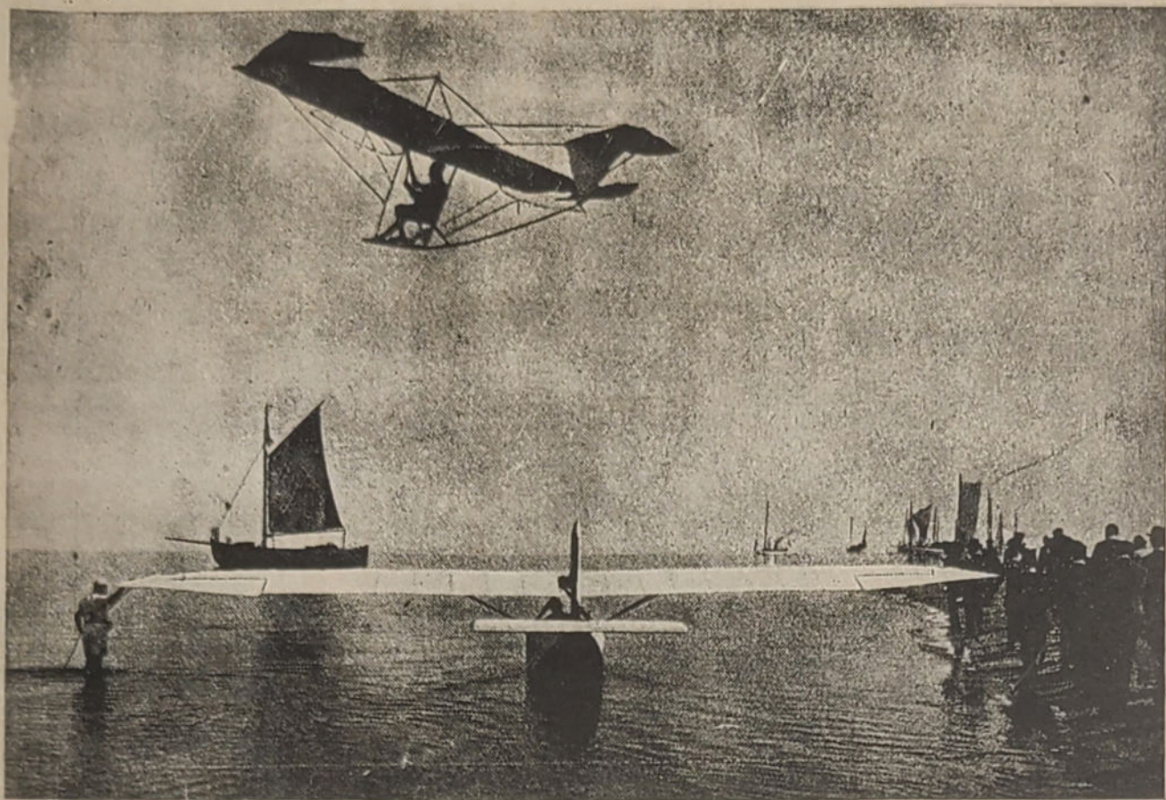
Un vuelo del avión de Schulz. En este momento está pasando sobre el hidroavión "Koenisberg", también sin motor
