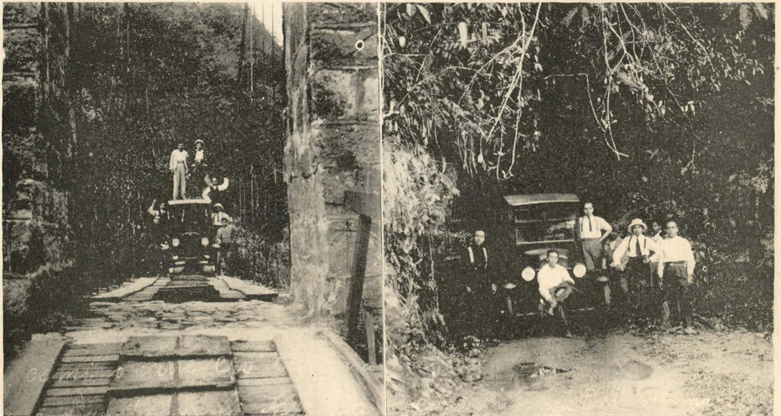
La fotografía de la izquierda se refiere al paso del camión "Overland Spad" por el puente de Herrería del camino carretero de Chanchamayo. La de la derecha corresponde al momento en que el "Overland Spad" continuando su viaje sale del túnel de Protolongo.
