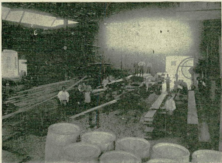
Una de las poderosas aserradoras de la Fábrica.
