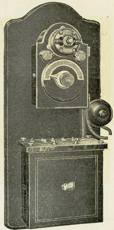
El Cronómetro eléctrico VICTOR, que mide automáticamente la duración de las exposiciones radiográficas.
