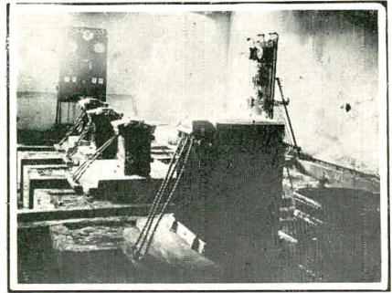
Sección de electricidad de la Escuela de Artes y oficios - Sala de transformaciones.
