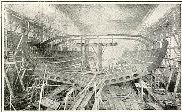
Construcción del gran acorazado francés «Jean Bart»
