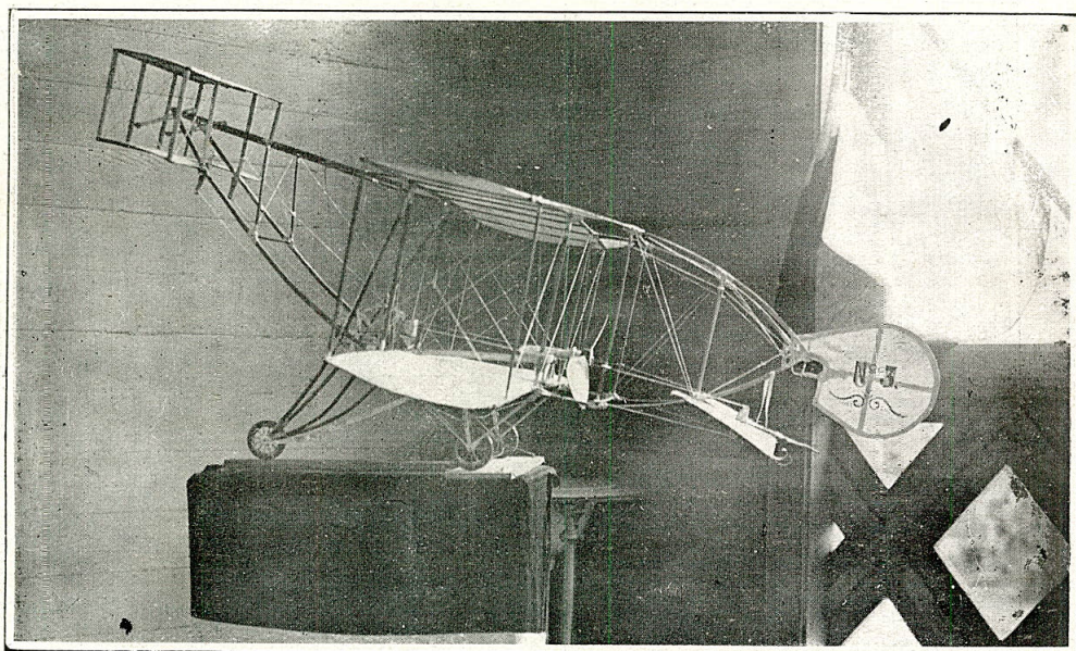
Modelo del aeroplano del mecánico Solórzano
