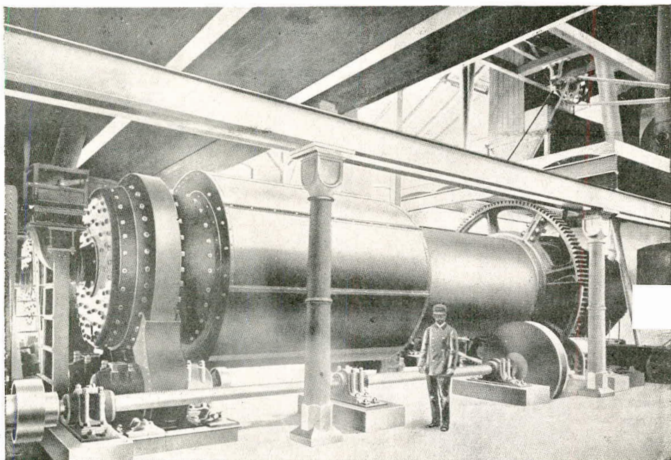
Máquina para moler el cemento y las materias primas.
