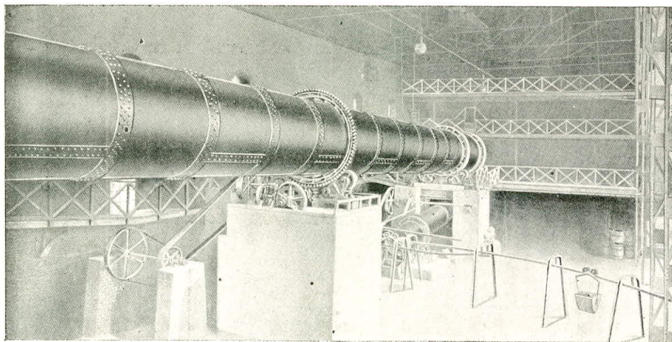
Tipo de la instalación del horno rotatorio, enfriadera y transportador del Clinker (Cemento quemado en fragmentos gruesos antes de ser molido), que para la manufactura del cemento Portland, implantará la Compañía en su fábrica de Lima.
