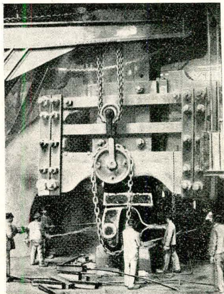
El martillo pilón de la casa Krupp que provee de cañones á los ejércitos de Alemania.
