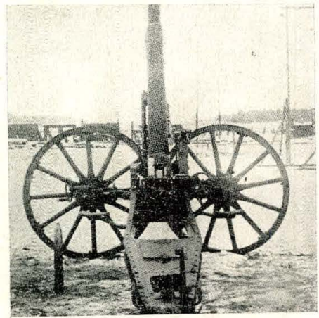
Cañón especial de los alemanes contra aeroplanos. (El cable nos ha anunciado que el cañón contra aeroplanos de los alemanes es formidable).
