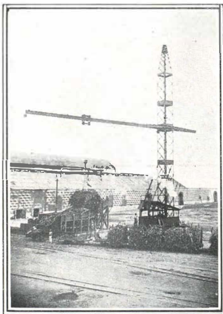
Hacienda "Roma". Grúa para descargar la caña al conductor.
