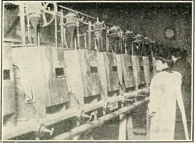
Batería de sopletes para la fabricación artificial de zafiros en el taller Disciyn, de Boulogne-sur-Seine, cerca de París
