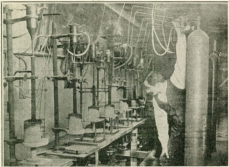
Fabricación artificial de rubíes en el taller Alexandre, en Sarcelles (Seine-et-Oise)
