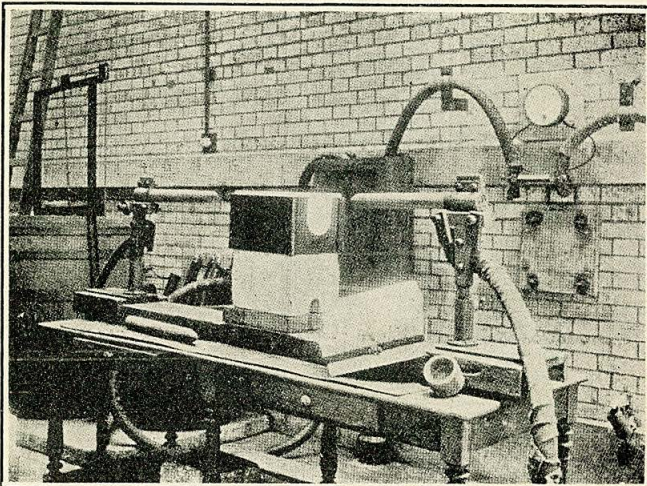
Horno eléctrico Moissan para realizar la síntesis del diamante
