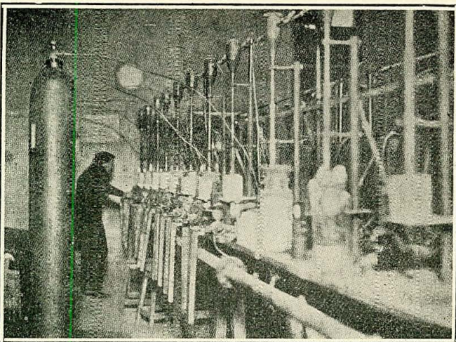
Puesta en marcha de los sopletes para la fabricación de los zafiros
