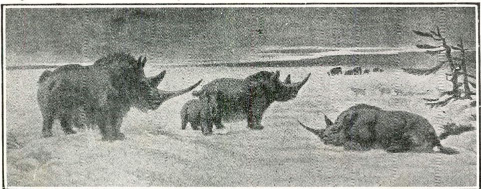
El invierno en el Norte de Francia durante los tiempos paleolíticos
